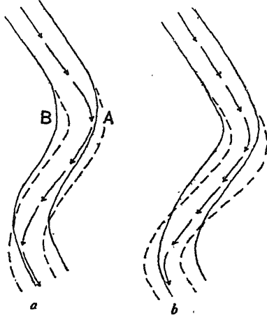
चित्र १५५—मिऐन्डर्स के निर्माण की विभिन्न दशायें।
